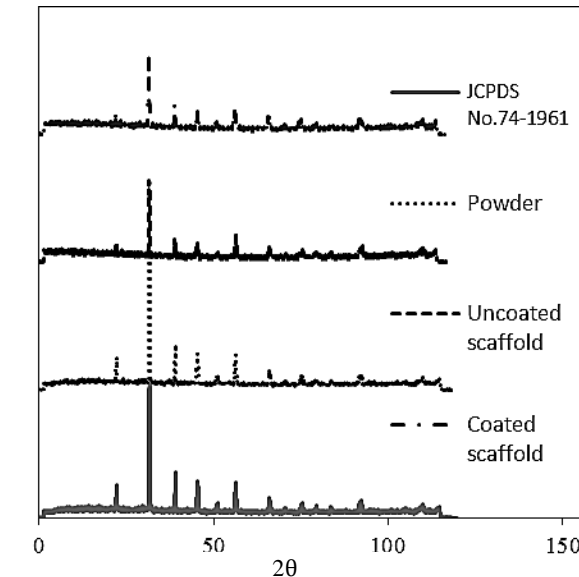
Fig. 6 XRD charts
